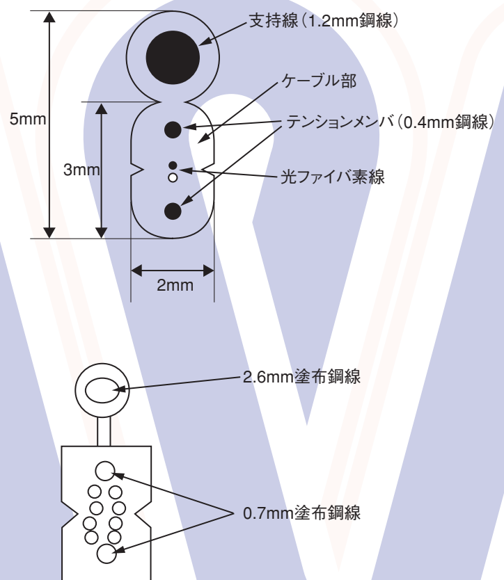
光ドロップワイヤー断面図事例
