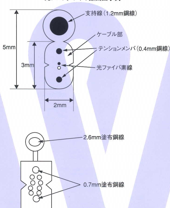
光ドロップワイヤー断面図事例
