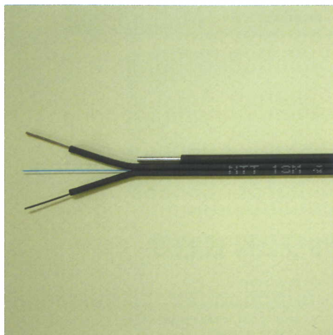
光ドロップワイヤー Fiber Optic Drop Cable
